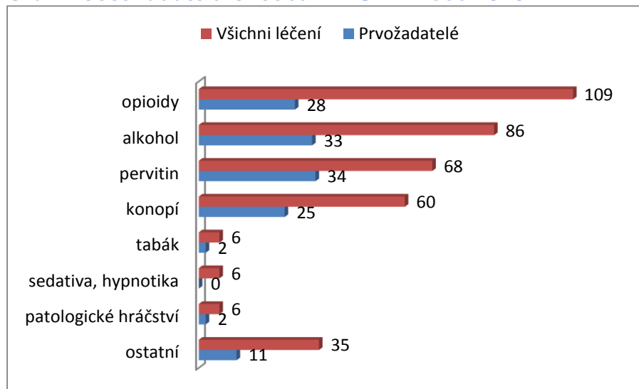
Graf Počet žadatelů o léčbu v MSK v roce 2016
