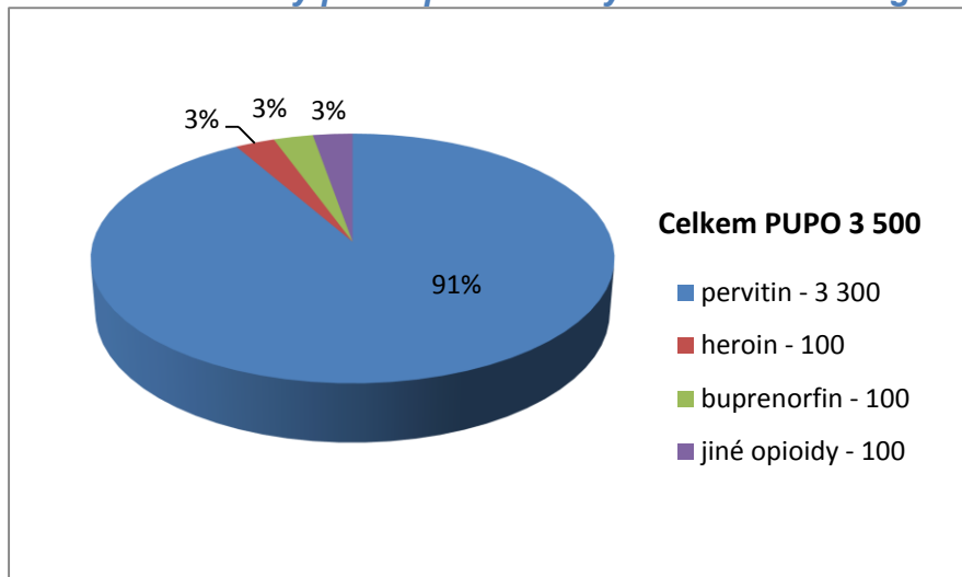
Graf Odhadovaný počet problémových uživatelů drog v MS kraji v roce 2016
