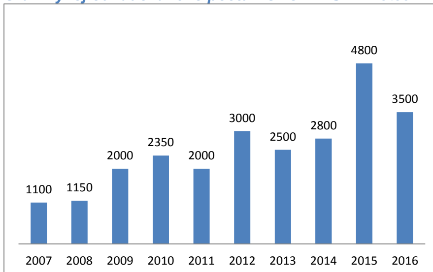
Graf Vývoj odhadovaného počtu PUPO v MSK v letech 2007 - 2016
